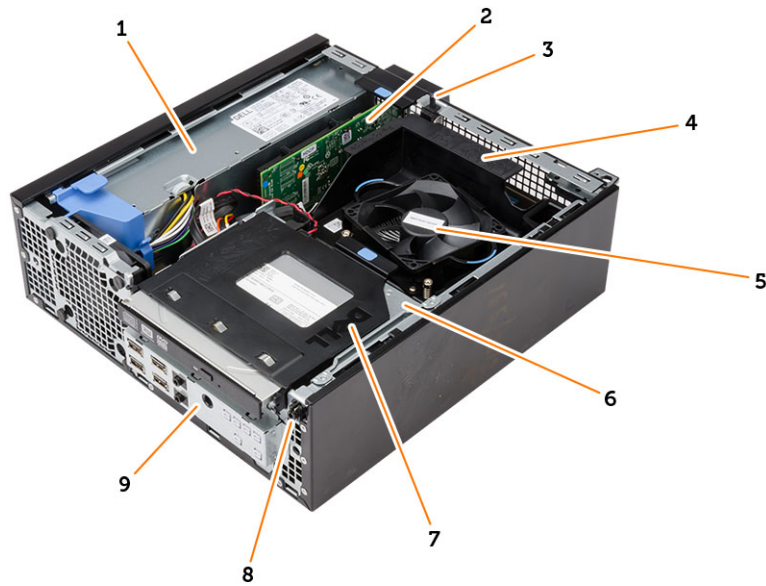
그림 2. 내부 모습
